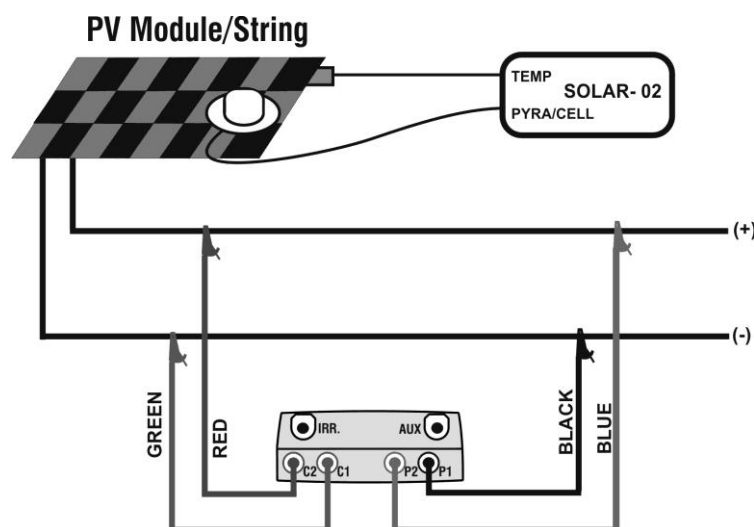
Fig. 9: Ligação do instrumento ao painel/bateria de painéis (stringa) FV
