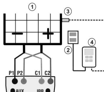
Fig. 15: Conexões do instrumento para testes IVCK com med. de Irrad./Temp com SOLAR-02
