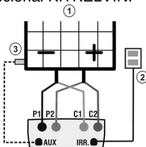
Fig. 14: Conexões do instrumento para testes IVCK com med. Direta de Irrad./Temp
