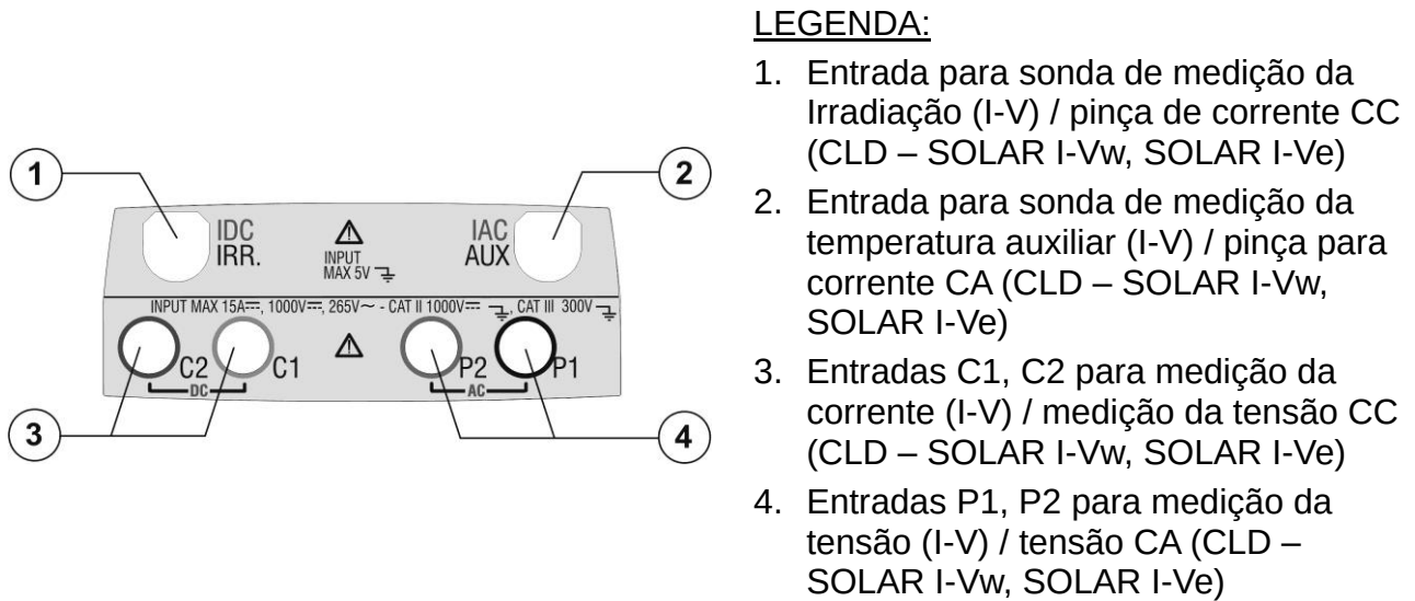
Fig. 2: Descrição da parte superior do instrumento
