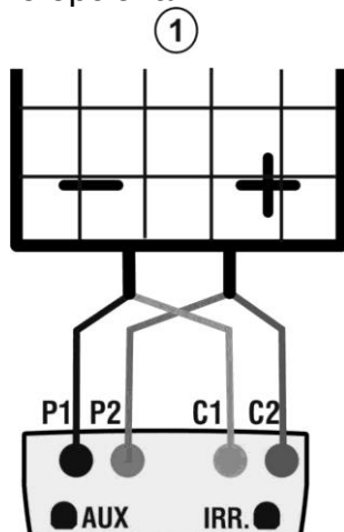
Fig. 13: Ligação ao painel/bateria FV para testes IVCK sem medição da Irradiação
