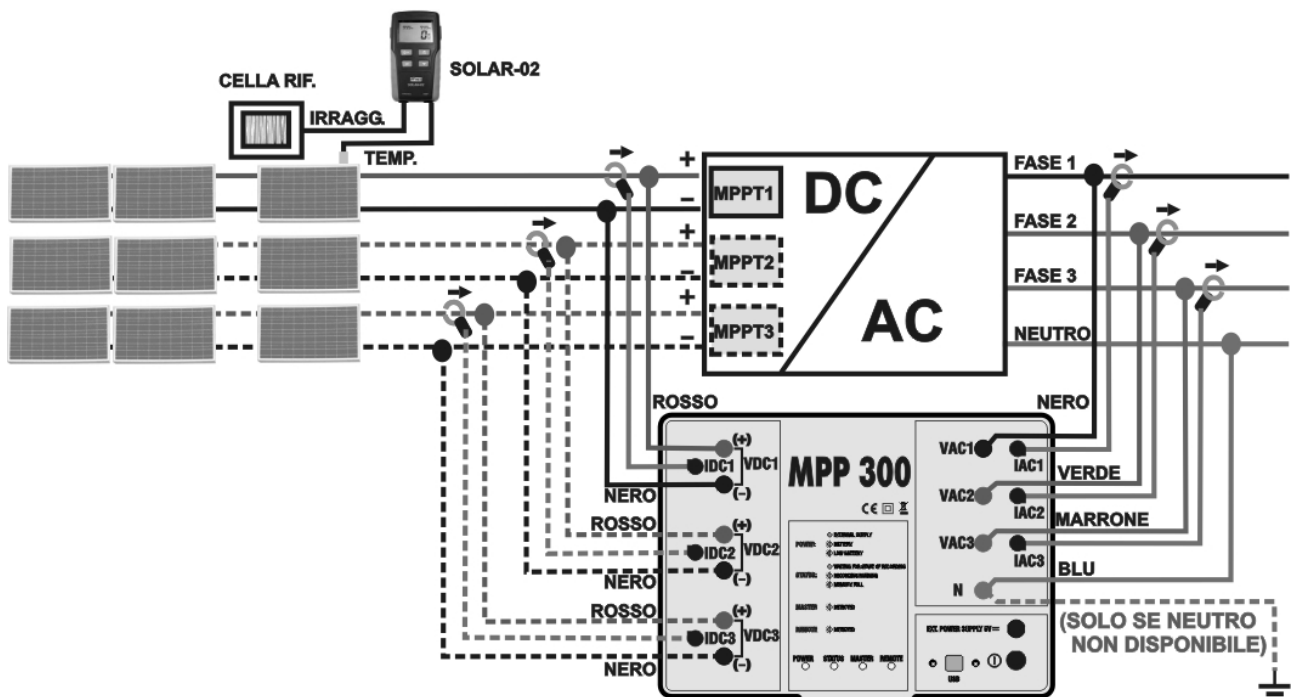
Fig. 6: Ligação do MPP300 para o teste de uma instalação FV Trifásica
