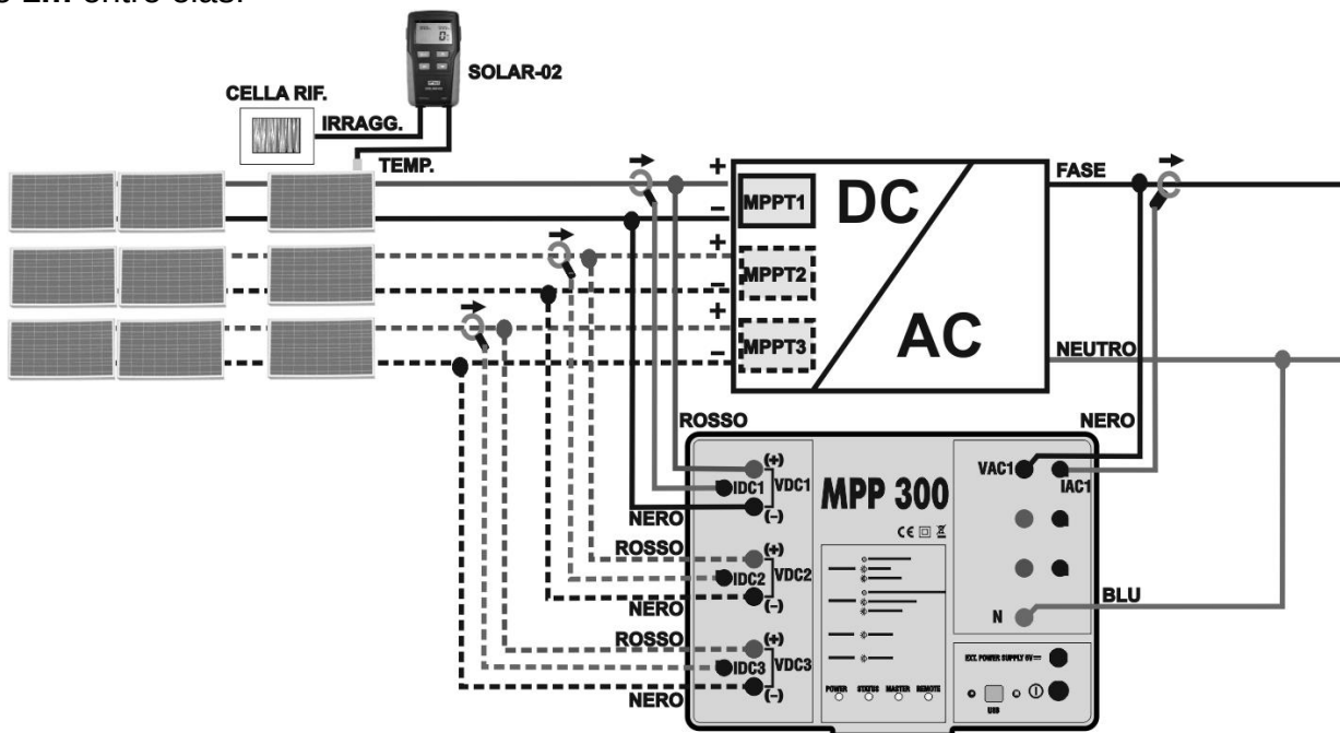
Fig. 5: Ligação do MPP300 para o teste de uma instalação FV Monofásica
