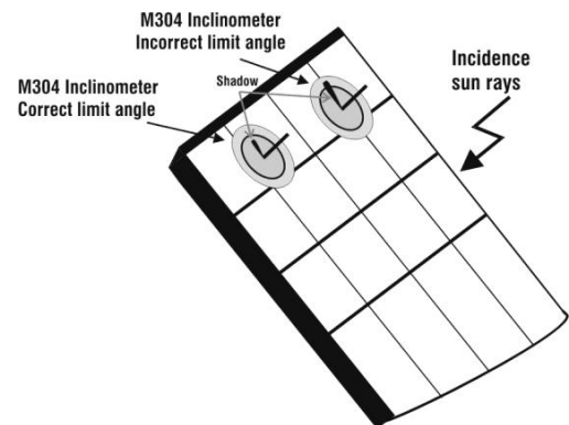
Fig. 7b: Colocação do inclinómetro M304
