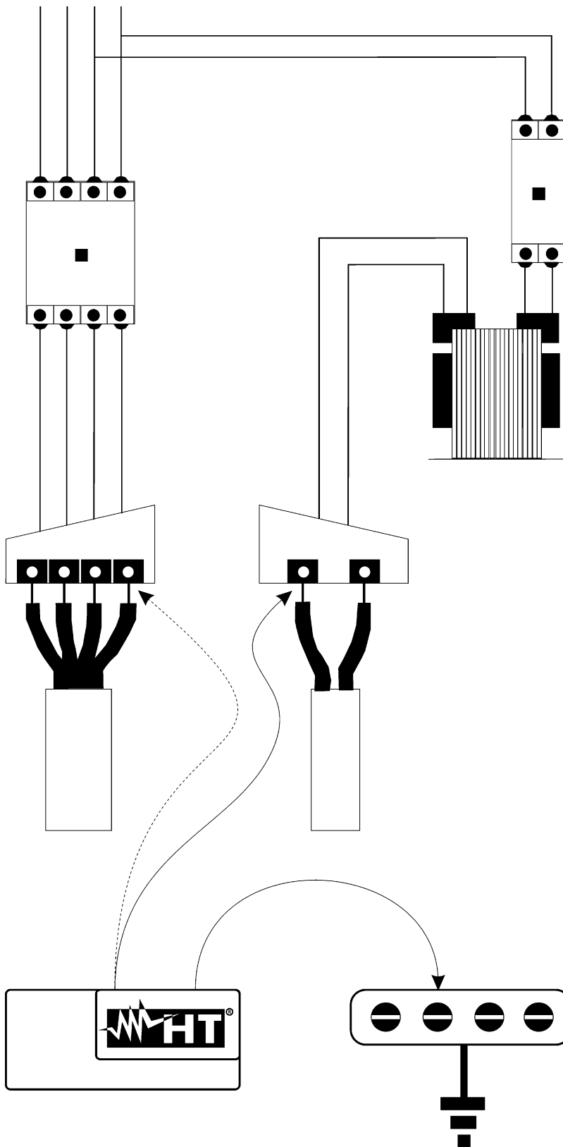
Fig. 44: Medidas de separação entre circuitos numa planta
