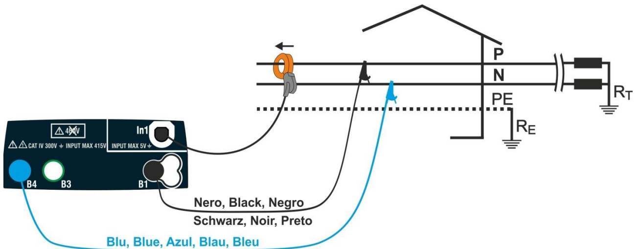
Fig. 42: Ligação para medição em sistema Monofásico
