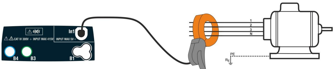
Fig. 37: Medição de corrente de fuga indireta em sistemas trifásicos
