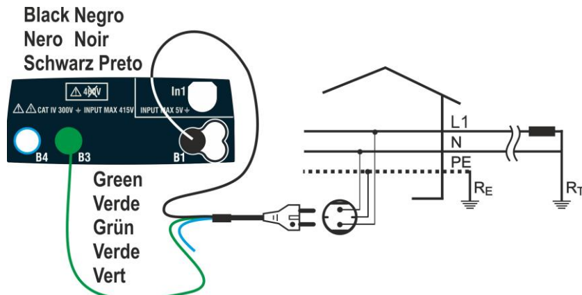
Fig. 31: Teste L1-PE de 2 fios para sistemas Monofásicos/Bifásicos com ficha Shuko
