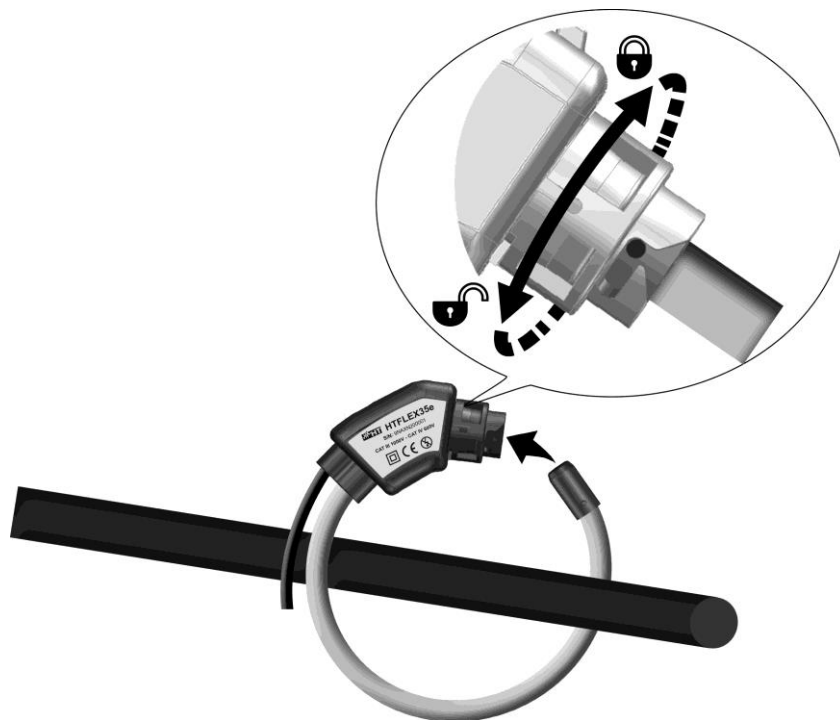
Fig. 3: Conexión de la pinza HTFLEX35e sobre el conductor
