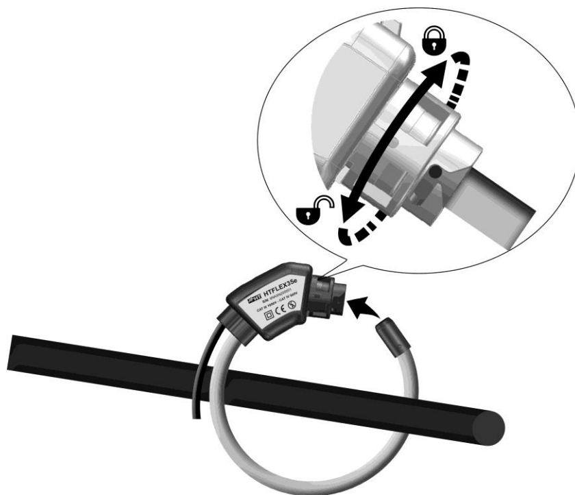
Fig. 3: Collegamento della pinza HTFLEX35e sul conduttore
