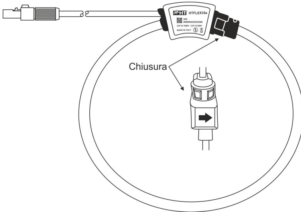
Fig. 2: Descrizione della pinza HTFLEX35e
