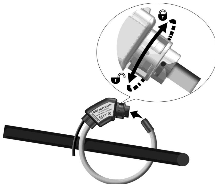
Fig. 3: Collegamento della pinza HTFLEX33e sul conduttore
