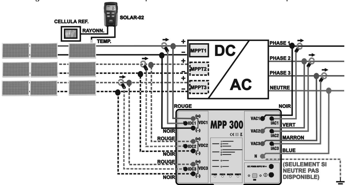
Fig. 6 : Connexion du MPP300 pour essai d'une installation PV Triphasée
