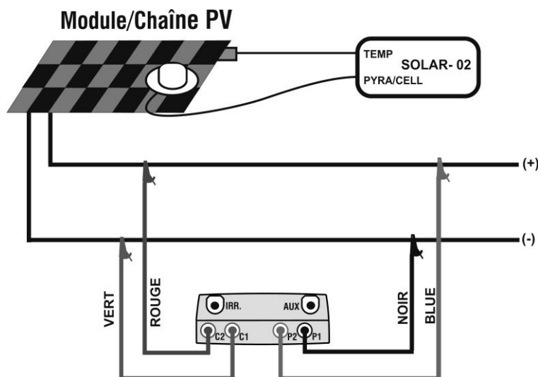
Fig. 9 : Connexion de l'instrument au module/chaîne PV
