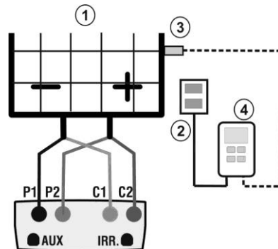
Fig. 15 : Connexions de l'instrument pour essais IVCK avec mes. de Rayonn./Temp par SOLAR-02
