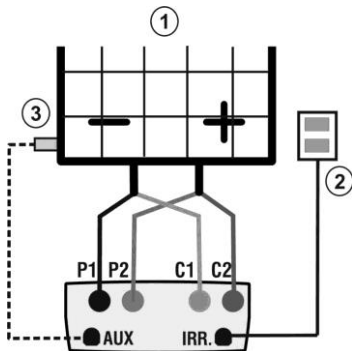
Fig. 14 : Connexions de l'instrument pour essais IVCK avec mes. directe de Rayonn./Temp
