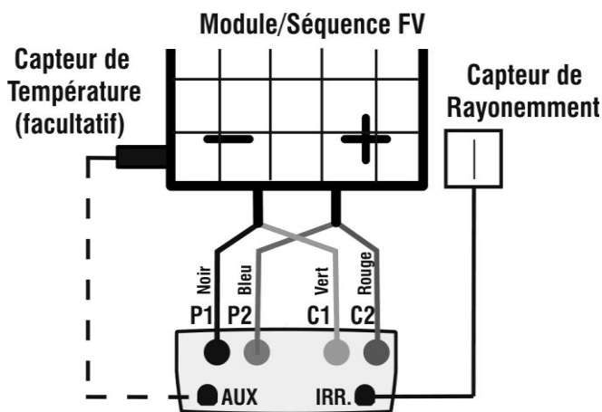
Fig. 7a : Connexion de l'instrument au module/chaîne PV M304
