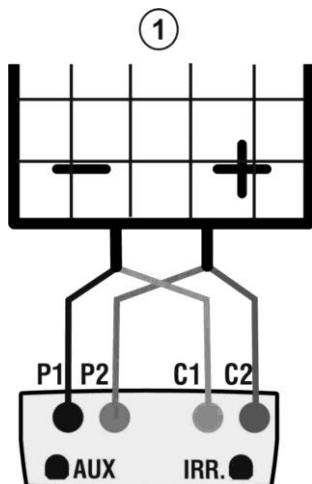
Fig. 13 : Conn. instrument au module/chaîne PV pour essais IVCK sans mesure rayonn.
