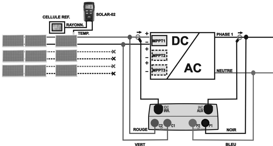
Fig. 4 : Connexion de l'instrument pour essai sur une installation PV Monophasée
