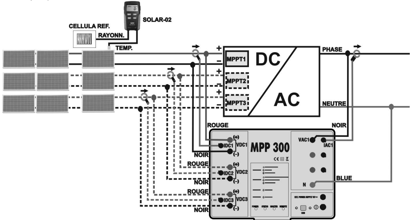
Fig. 5 : Connexion du MPP300 pour essai d'une installation PV Monophasée
