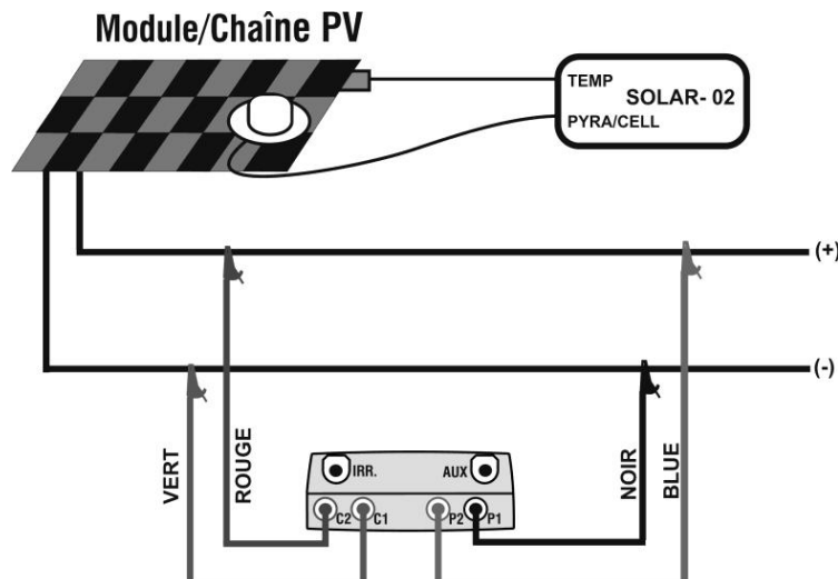
Fig. 11 : Connexion de l'instrument au module/chaîne PV
