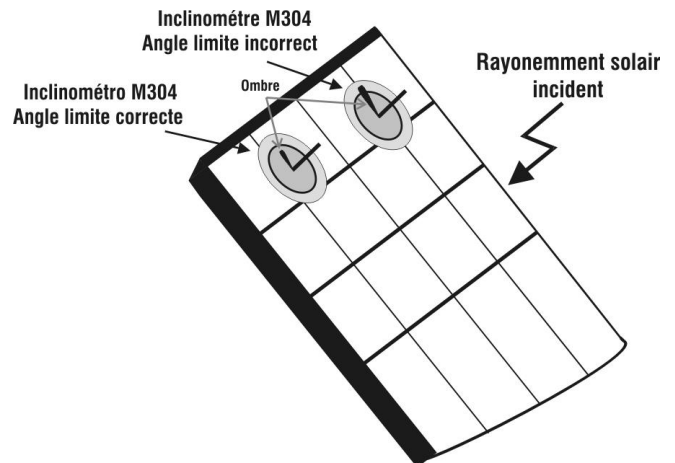
Fig. 7b : Positionnement inclinomètre
