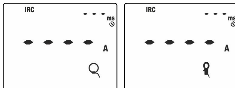
Fig. 40 : Pages-écrans initiales de mesure du courant de démarrage
