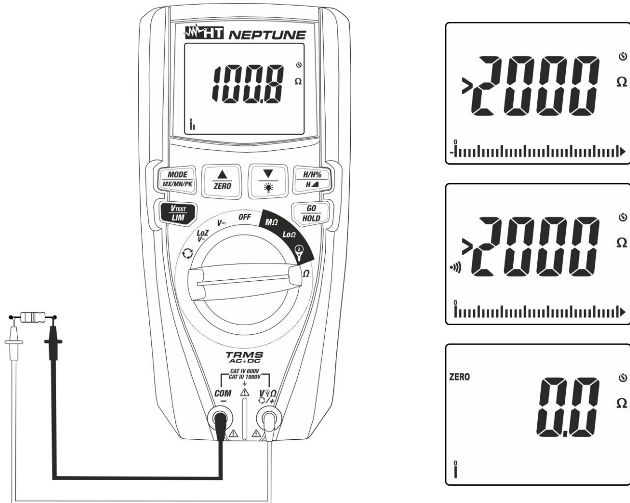
Fig. 9: Utilisation de l'instrument pour mesure de résistance et test de continuité
