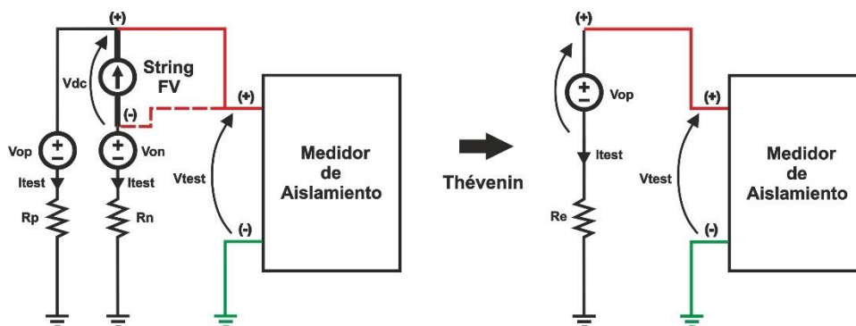
Fig. 10: Diagrama y circuito equivalente del Método 1
