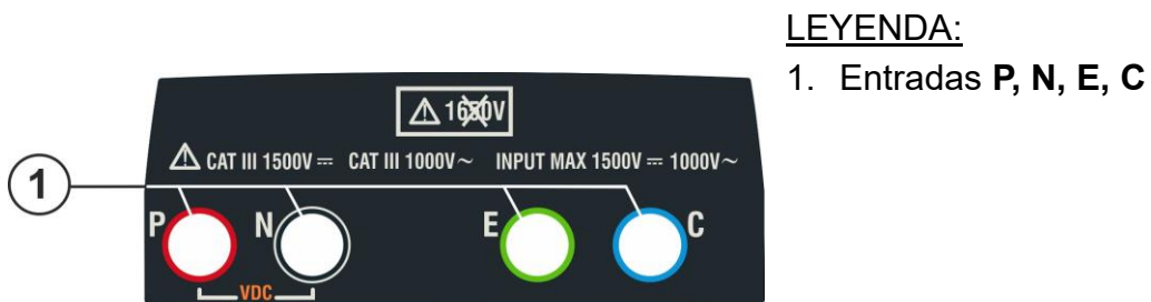
Fig. 1: Descripción parte frontal del instrumento
