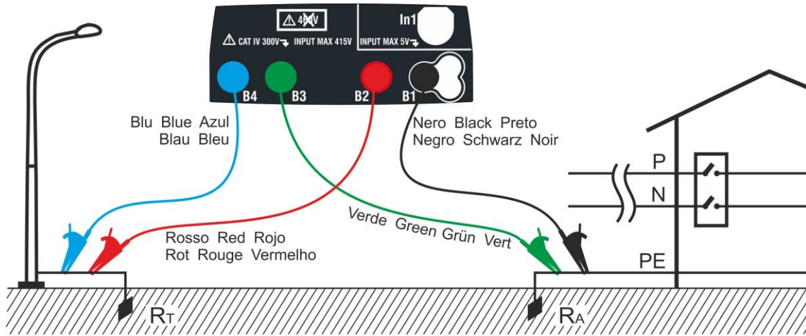
Fig. 29: Medida de la resistencia de tierra a 2 hilos con dispensador auxiliar
