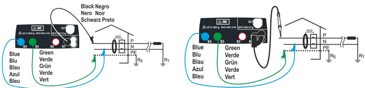
Fig. 13: Conexionado en sistema monofásico 230V con cables y punta remota
