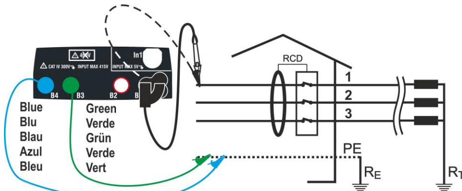
Fig. 16: Conexión en sistema trifásico 400V+ PE (no N) con cables y punta remota (no para RCD tipo B)
