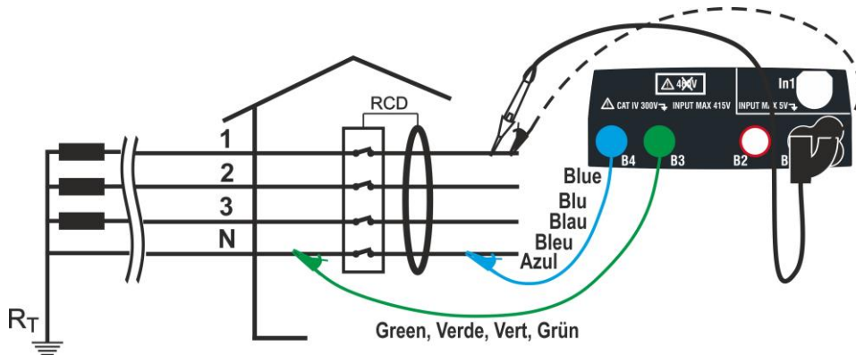
Fig. 15: Conexión 400V+ N (no PE) con cables y punta remota
