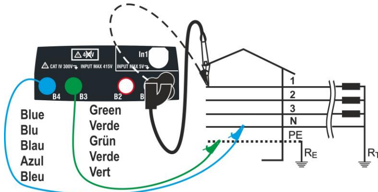
Fig. 23: Medida P-PE en sistemas IT con cables y punta remota
