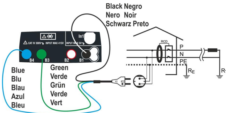
Fig. 12: Conexionado en sistema monofásico 230V mediante la toma shuko
