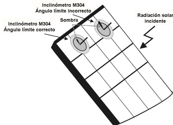
Fig. 10: Posicionamiento inclinómetro M304 Módulo/Grupo módulos FV
