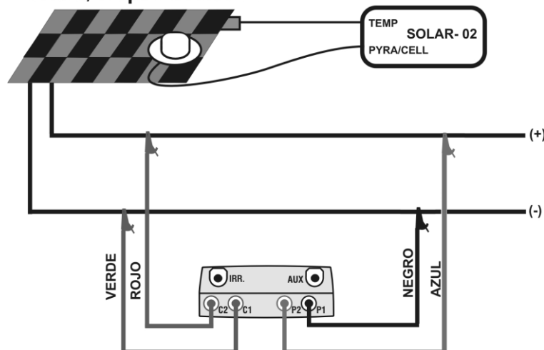
Fig. 11: Conexión del instrumento al módulo/stringa FV
