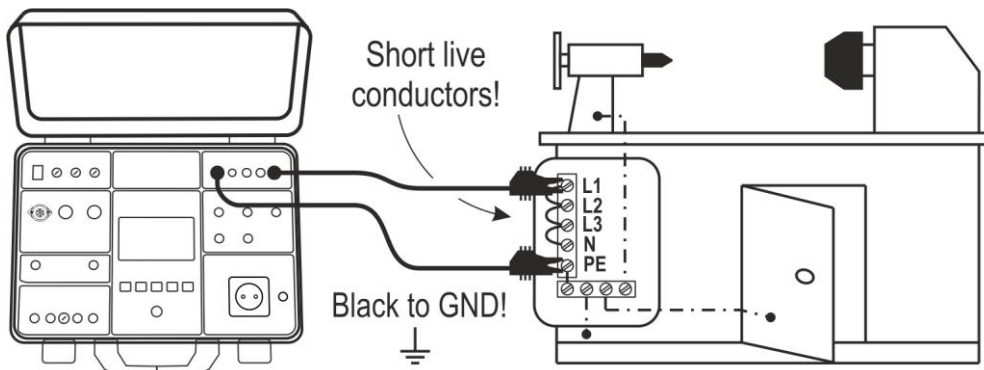
Fig. 39: Conexión de las puntas de prueba por el test DIELECTRIC
