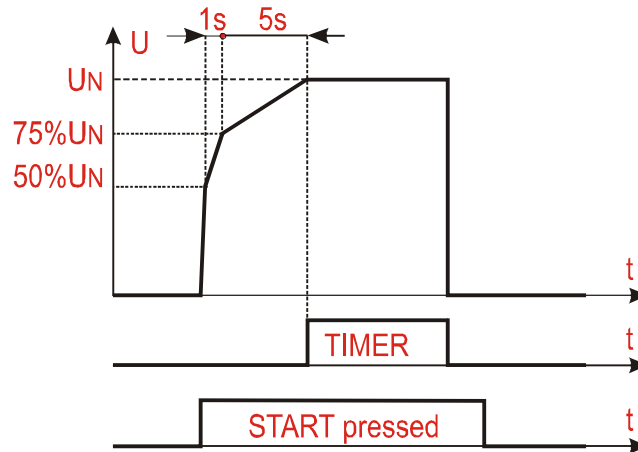
Fig. 38: Prueba DIELECT en modos Rampa 50%
