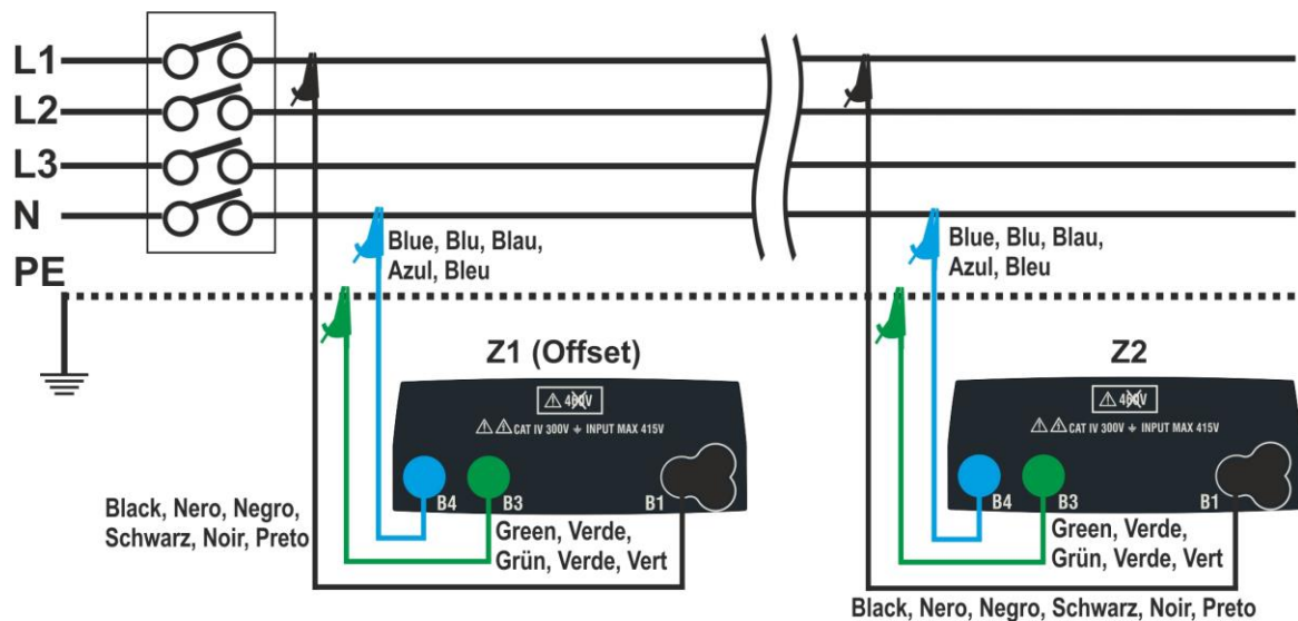
Fig. 37: Conexión del instrumento para la medida de la caída de tensión modo L-N
