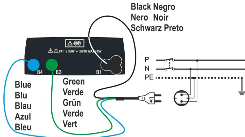
Fig. 8: Conexión del instrumento con toma de corriente
