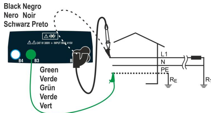
Fig. 32: Prueba L1-PE 2-hilos para sistemas Monofásicos/Bifásicos con cables y punta remota remota
