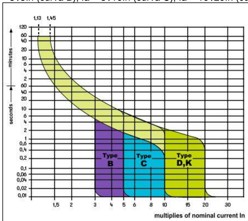
Fig. 41: Ejemplo de curvas relativas a la protección magnetotérmica (MCB)
