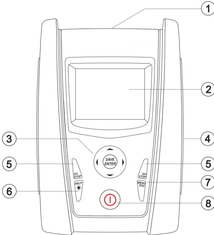
Fig. 1: Descripción del frontal del instrumento
