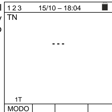
Fig. 36: Verificación de la secuencia de fase con punta remota
