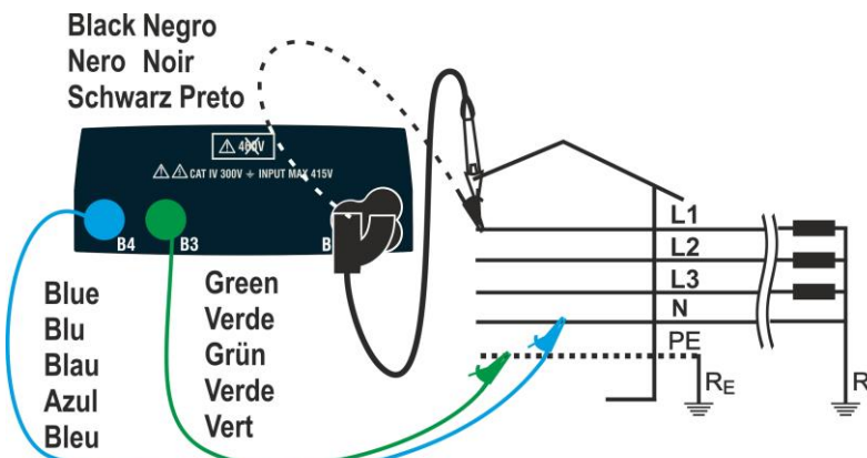
Fig. 27: Prueba L-N/L1-PE para sistema Trifásico con cables y punta remota
