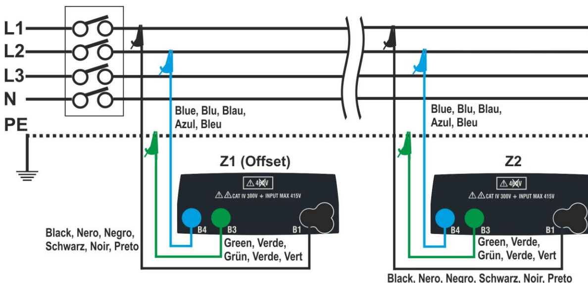
Fig. 38: Conexión del instrumento para la medida de la caída de tensión modo L-L
