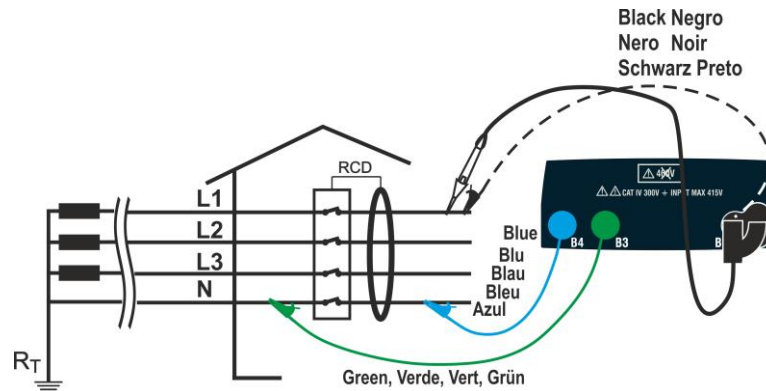
Fig. 23: Conexión para sistema Trifásico L1,L2,L3,N (sin PE) con cables y punta remota
