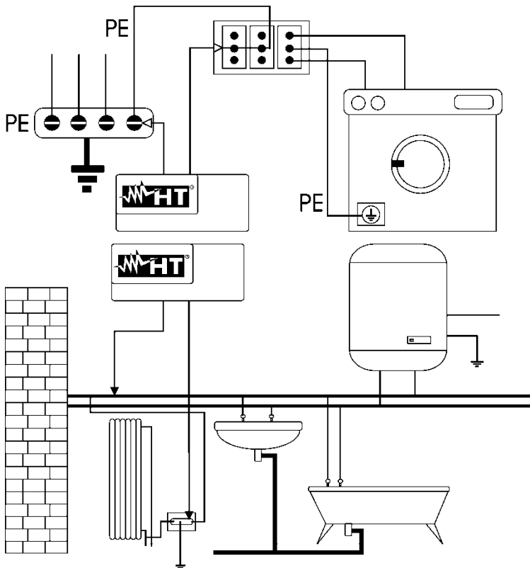
Fig. 39: Ejemplos de medida de continuidad de los conductores
