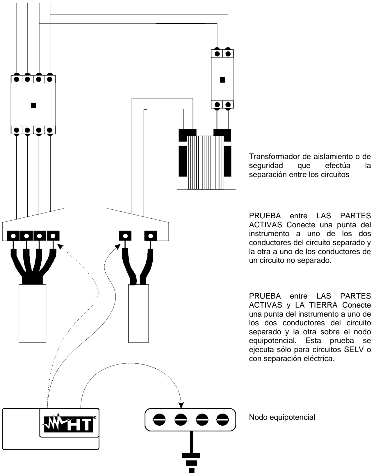
Fig. 40: medida de separación entre circuitos en una instalación
