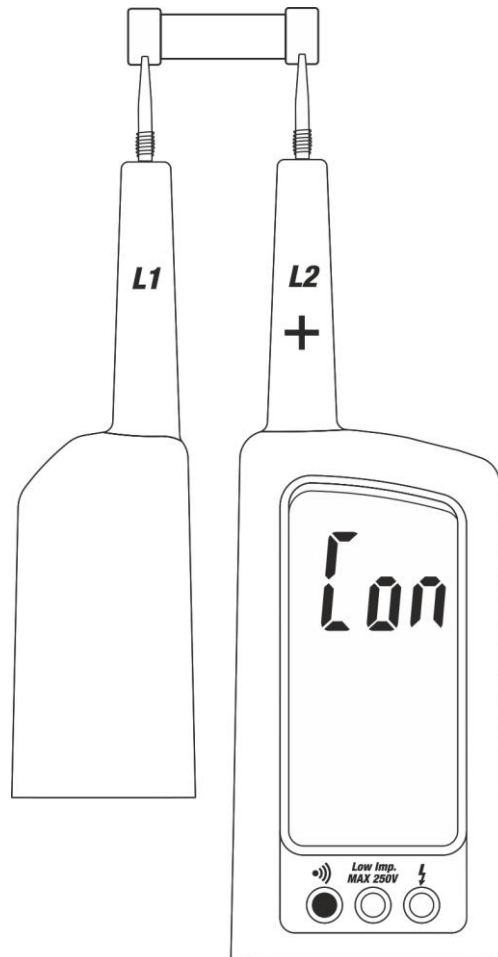
Fig. 7: Prueba de Continuidad
