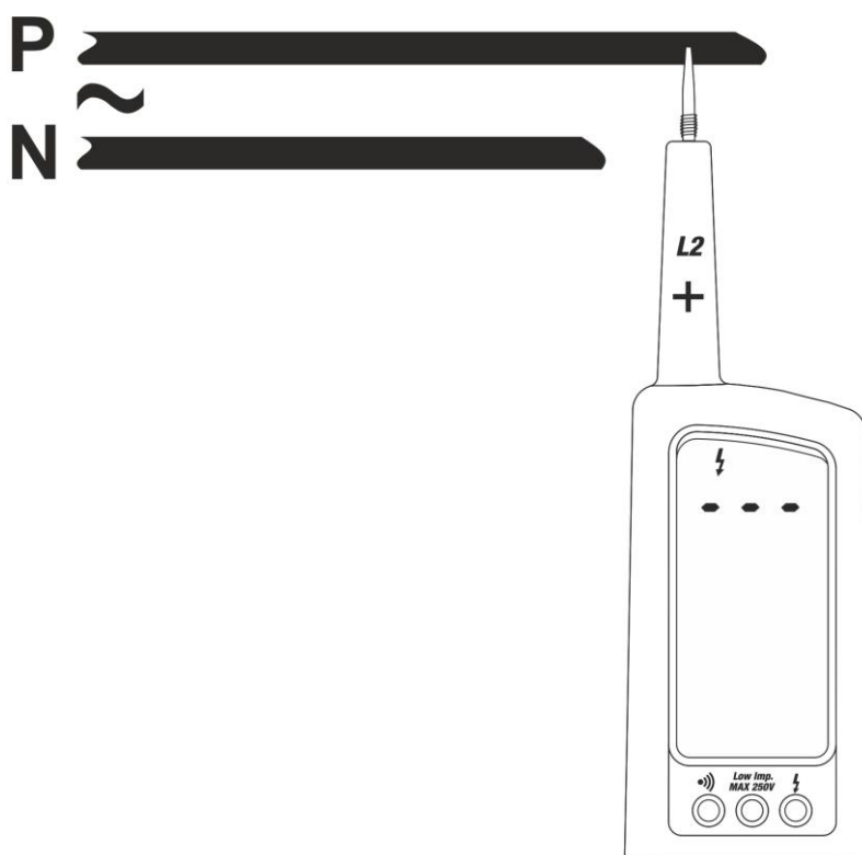
Fig. 5: Détection de Tension CA avec 1 fil
