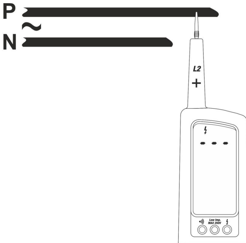
Abb. 5: Phasenprüfung einpolig
