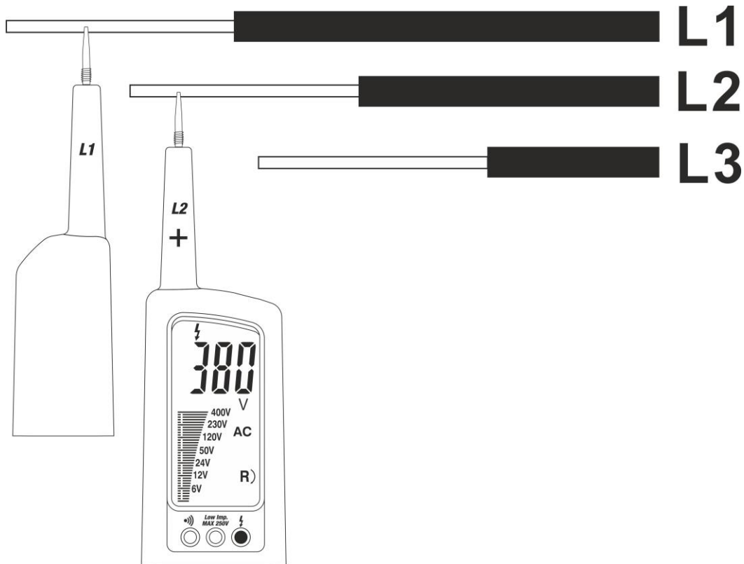
Fig. 6: Senso ciclico delle fasi
