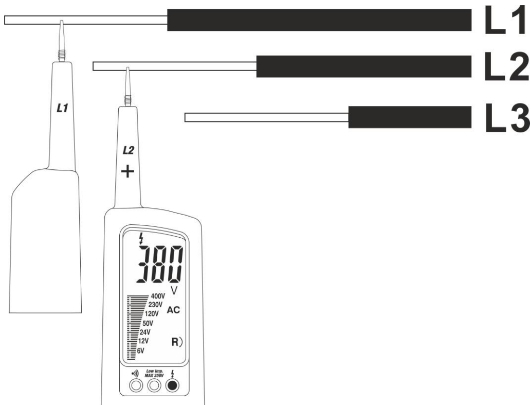
Fig. 6: Test rotation des phases
