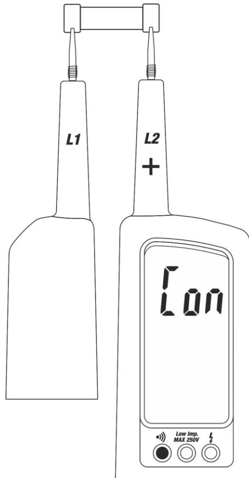
Fig. 7: Teste de Continuidade
