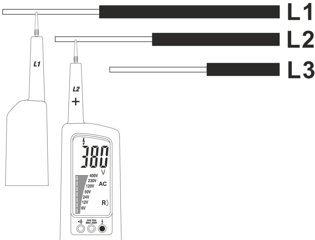
Fig. 6: Detección secuencia de fases
