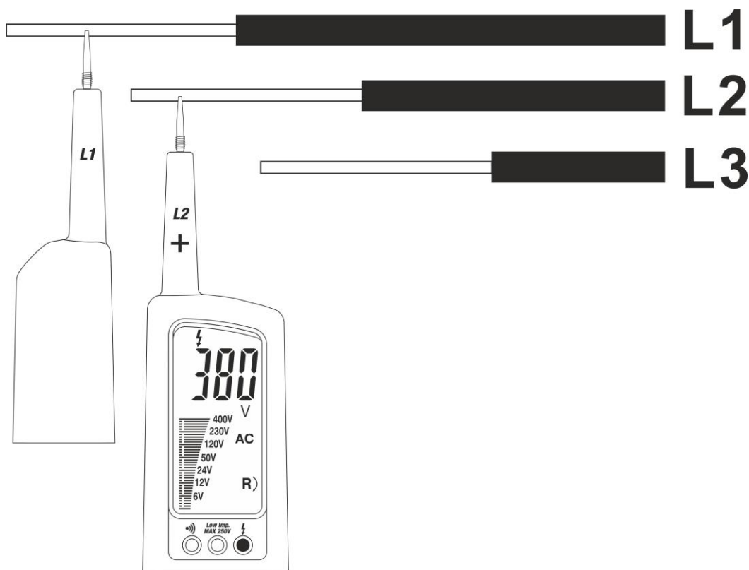
Fig. 6: Teste da sequência das fases
