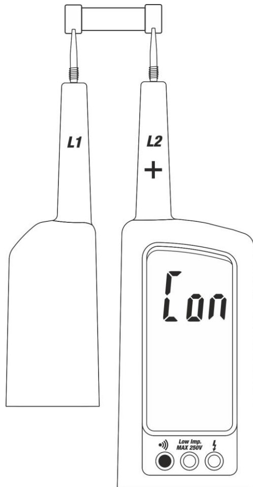
Fig. 7: Test Continuità
